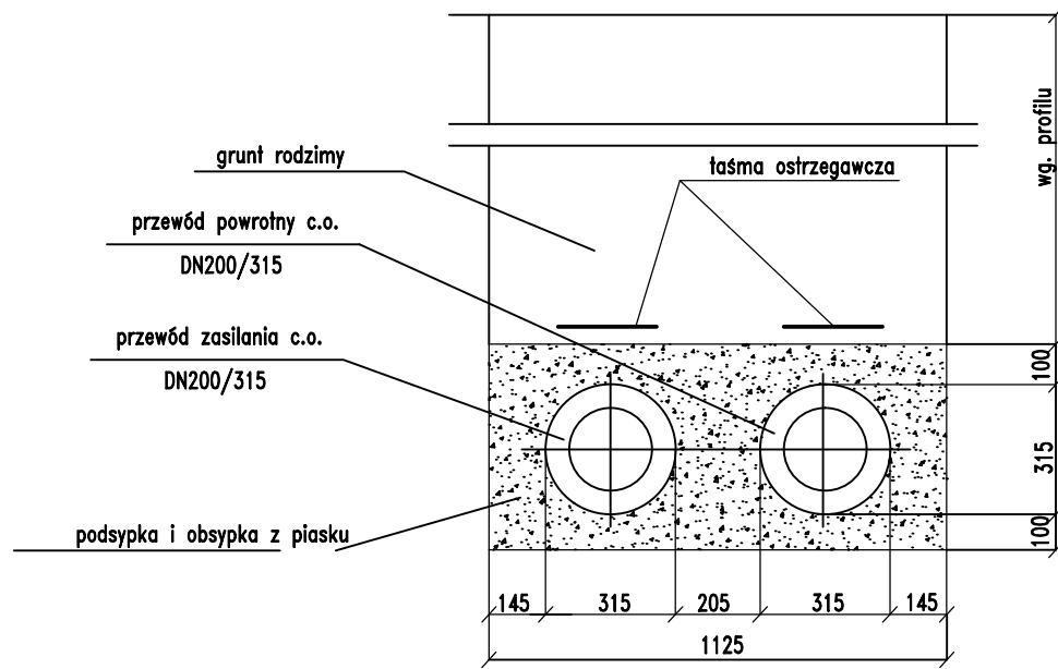
Przekrój wykopu, sieć ciepła 2xDN200/315
