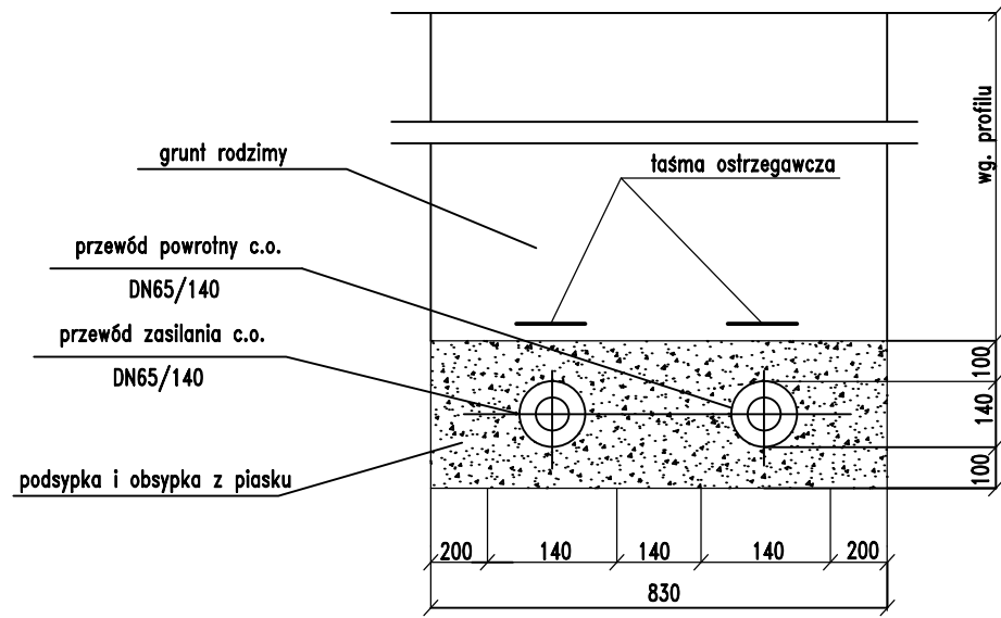
Przekrój wykopu, sieć ciepła 2xDN65/140
