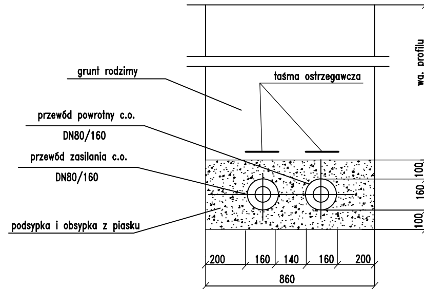
Przekrój wykopu, sieć ciepła 2xDN80/160
