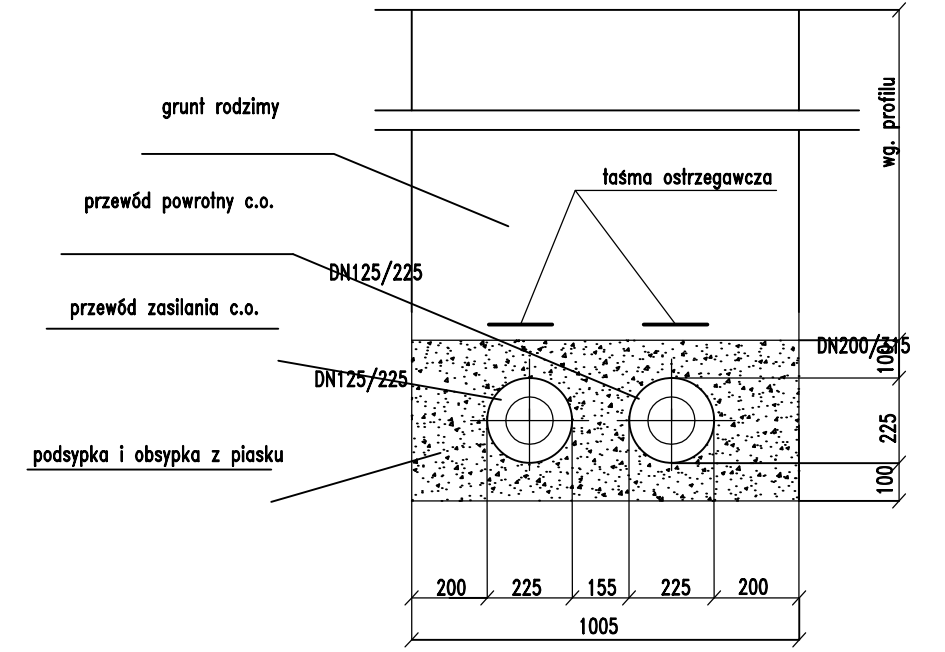
Przekrój wykopu, sieć ciepła 2xDn125/225
